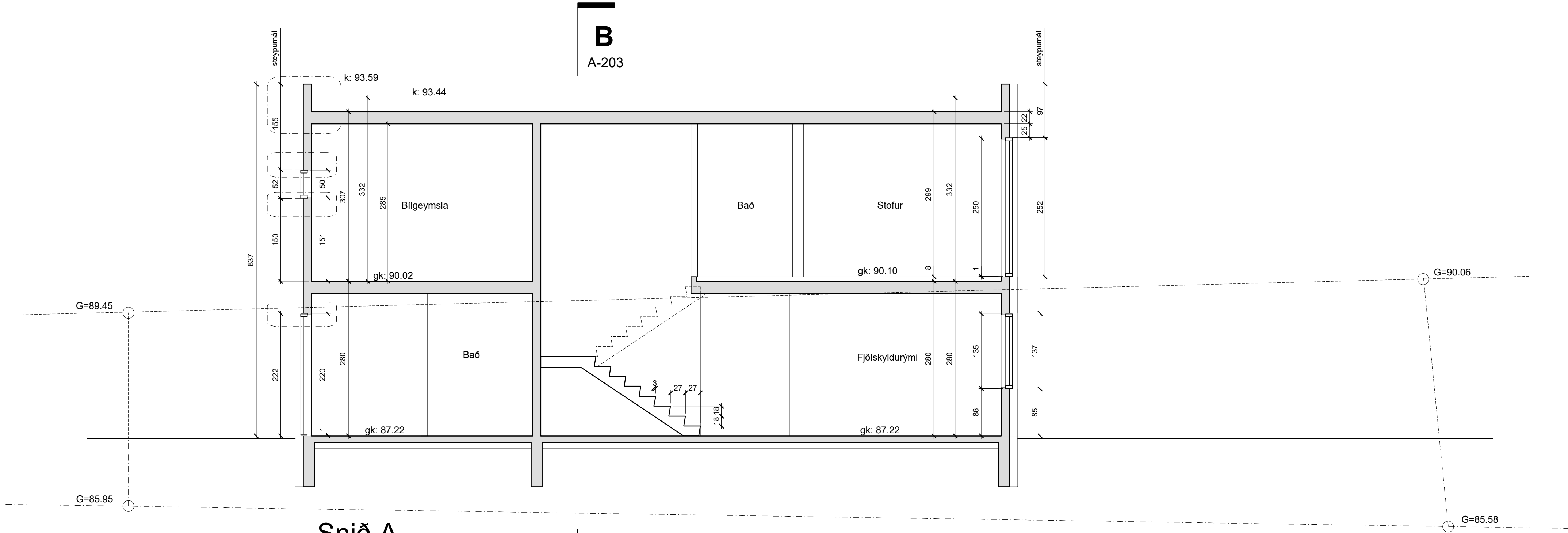
Snið A
