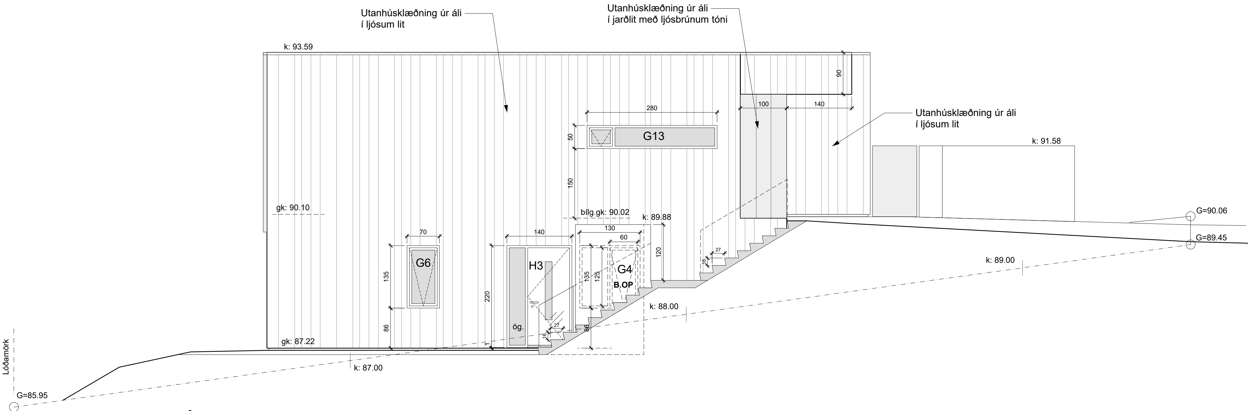
Útlit, norður
